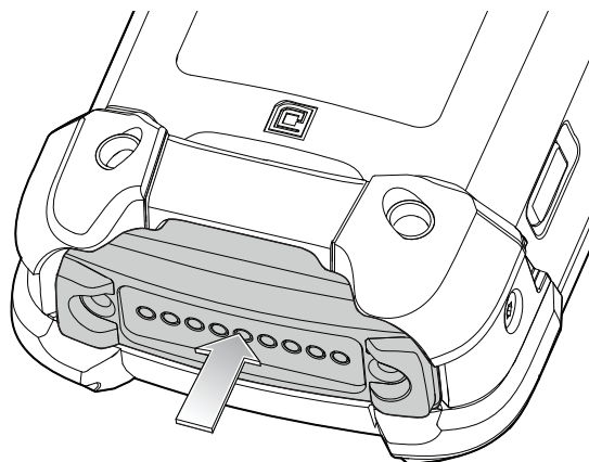
图 15 按入电池
