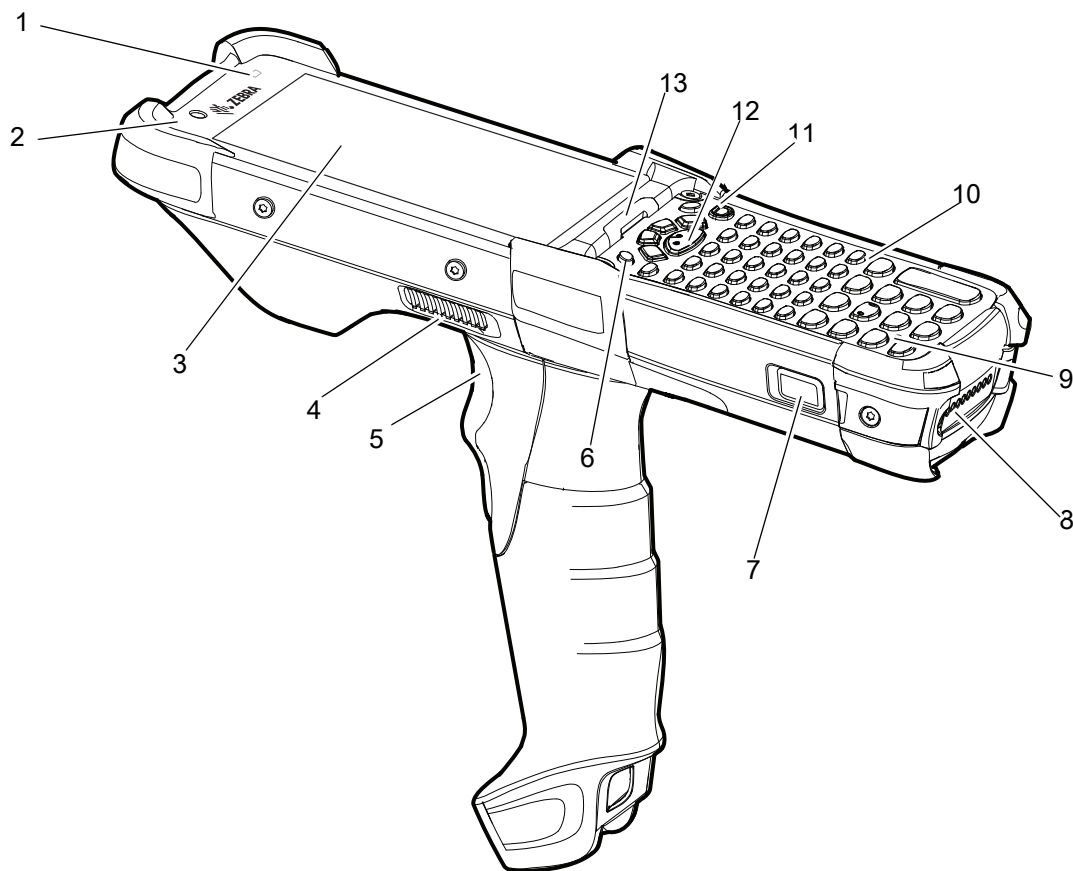
图 1 MC93XX 前视图
