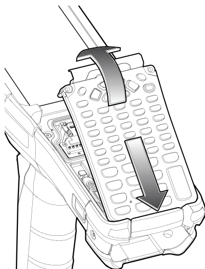
图 10 装回键盘
